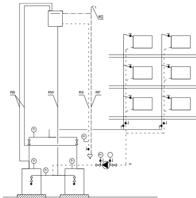
Rysunek 1b Schemat zabezpieczenia instalacji ogrzewania wodnego, wyposażonej w jeden kocioł lub wymiennik ciepła, rozdziel górnny, pompa zamontowana na powrocie wg PN-B-02414:1999.
