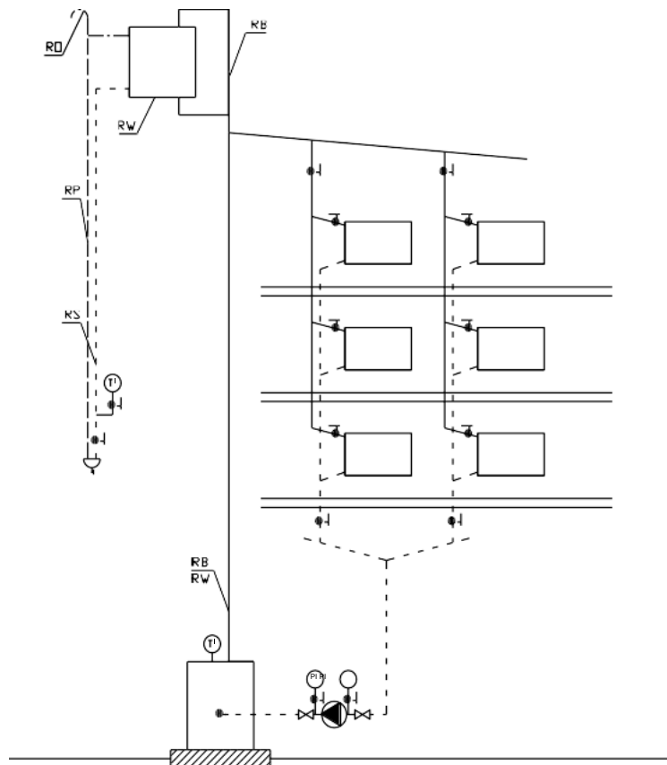
Rysunek 1b Schemat zabezpieczenia instalacji ogrzewania wodnego, wyposażonej w jeden kocioł lub wymiennik ciepła, rozdziel górnny, pompa zamontowana na powrocie wg PN-B-02414:1999.
