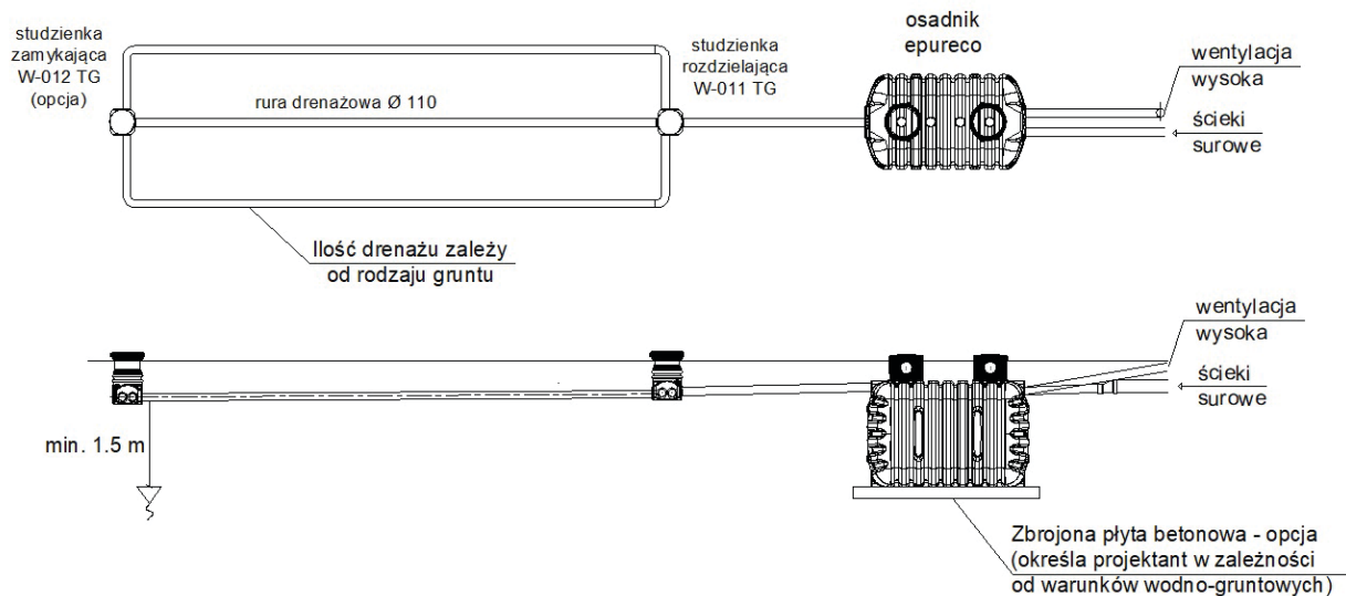
Przykładowy rzut i przekrój osadnika epureco z drenażem rozsączającym
