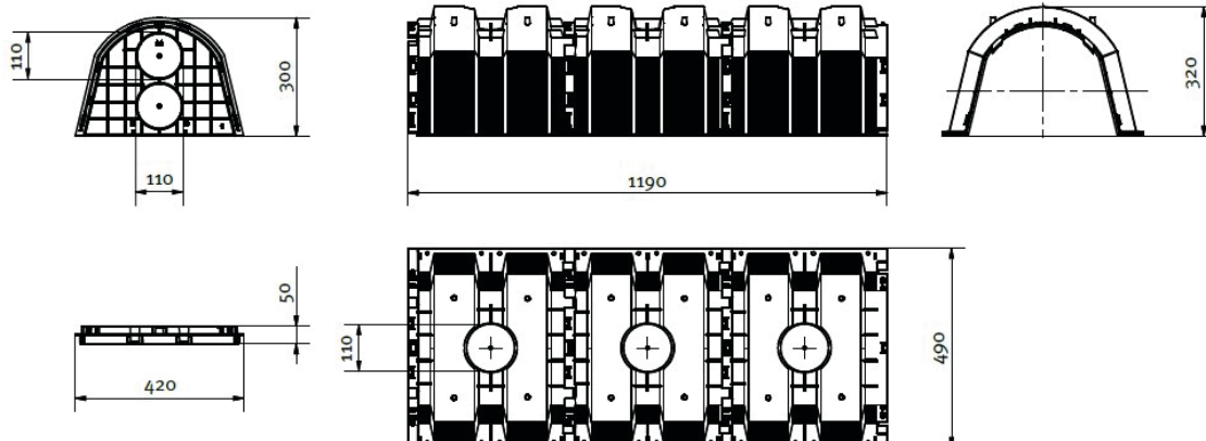
komora rozsączająca 130I – KOM-ST130 Dekiel ST – DEK-ST
