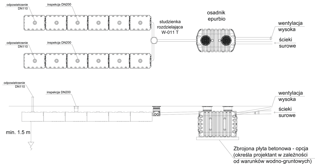
Przykładowy rzut i przekrój osadnika epurbio z tunelami rozsączaającymi
