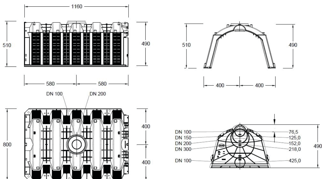
tunel rozsączający 300l – 230010 dekiel – 231004-S
