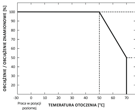
© CHARAKTERYSTYKA OBCIĄŻALNOŚCI W ZALEŻNOŚCI OD OBCIĄŻENIA
