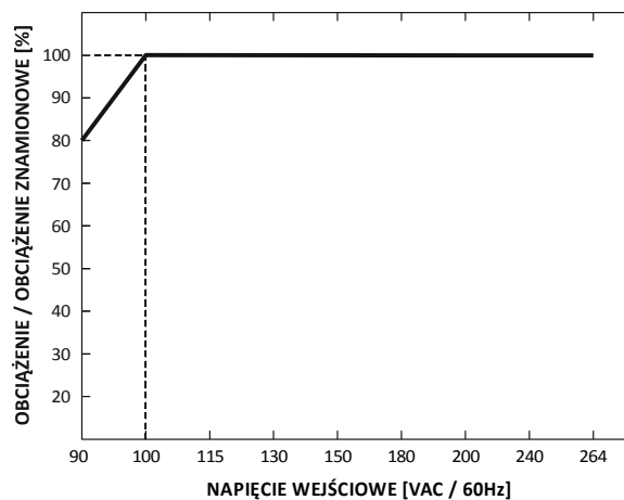
© CHARAKTERYSTYKA OBCIĄŻALNOŚCI W ZALEŻNOŚCI OD NAPIĘCIA WEJŚCIOWEGO
