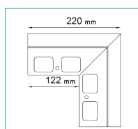
NZ K100/90 NAROŻNIK ZEWNĘTRZNY
