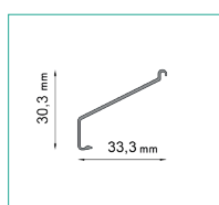
LK100 ŁĄCZNIK
