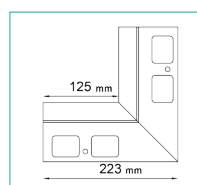
NW K100/90 NAROŻNIK WEWNĘTRZNY
