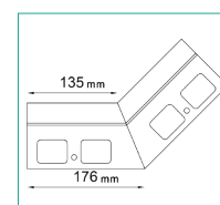
NW K100/135 NAROŻNIK WEWNĘTRZNY
