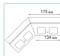
NZ K100/135 NAROŻNIK ZEWNĘTRZNY
