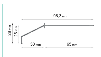
PROFIL PROSTY K100
