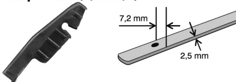
adaptor M1 (2,5 x 7,2)
