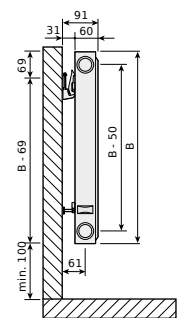
Compact, typ 11 z zawieszaniami ściennymi SSMS, widok z boku
