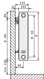
Compact, typ 22 z zawieszaniami ściennymi, widok z boku
