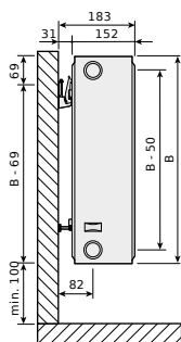
Compact, typ 33 z zawieszaniami ściennymi SSMS, widok z boku
