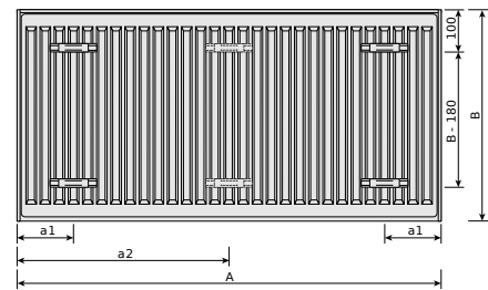
Compact, widok z tyłu (typ 21s, 22, 33)
