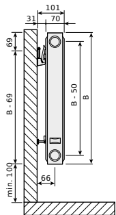
Compact, typ 21s z zawieszaniami ściennymi SSMS, widok z boku
