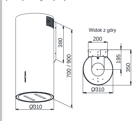
Rys. 2 Rysunek gabarytowy.
