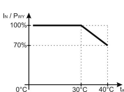
Wykres 1. Dopuszczalny prąd wyjściowy zasilacza w zależności od temperatury otoczenia (obciążenie chwilowe).
