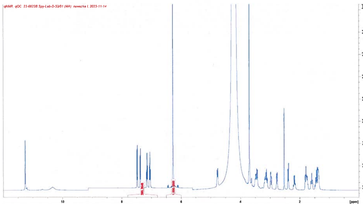
Widmo ^1\text{H} qNMR, Chlorowodorek johimbiny CAS: 65-19-0 (23-6623B), kwas maleinowy (Spy-Lab-D-53/01) w \text{DMSO-d}_6 .
