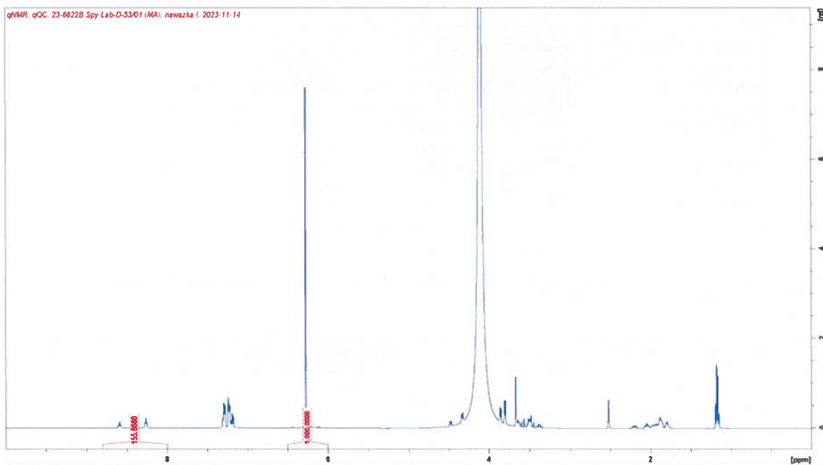
Widmo ^1\text{H} qNMR, noopept CAS: 157115-85-0 (23-6622B), kwas maleinowy (Spy-Lab-D-53/01) w \text{DMSO-d}_6 .
