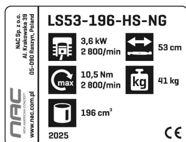
Tabliczka znamionowa
