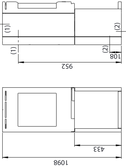
Jotul F 134 (na podstawie, bez szyb bocznych)
