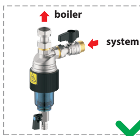
Rys 1. Rekomendowane miejsce montażu: OPCJA A
