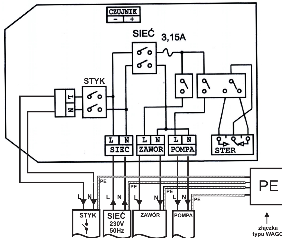
Rys. 2 Schemat elektryczny
