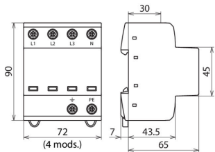
Rysunek wymiarowy DSH TNS 255
