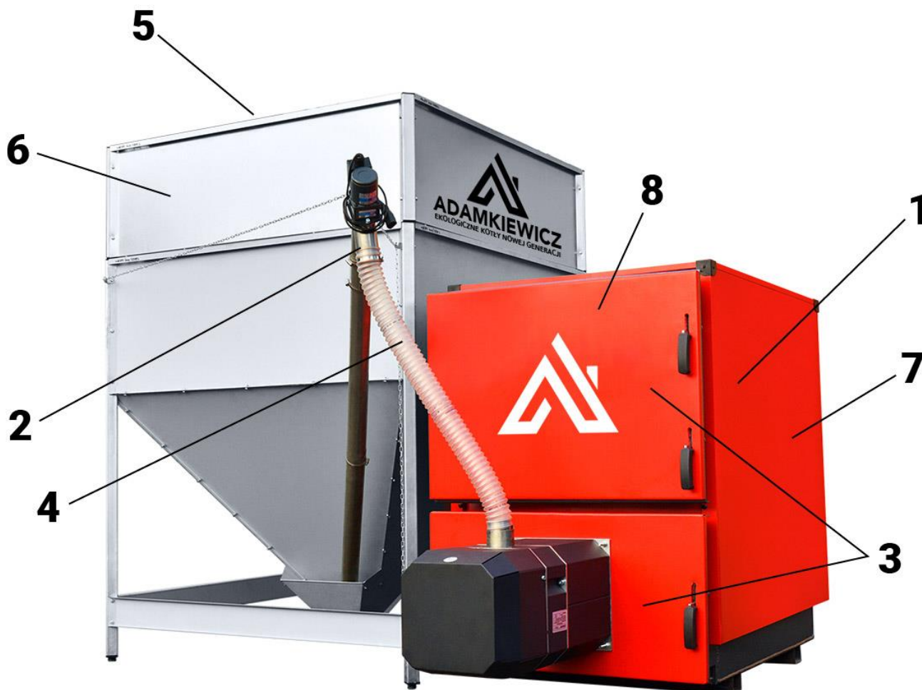
Rysunek 2. Budowa kotła PELLAR.
