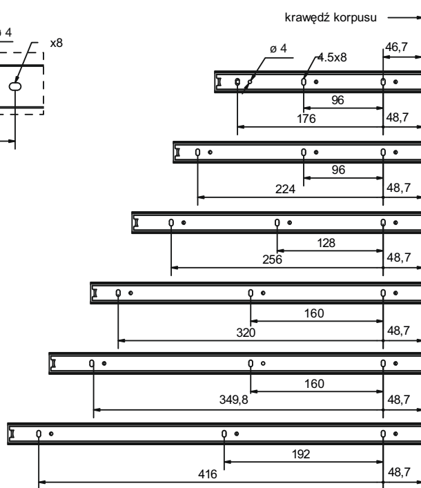
Widok na boku szuflady
