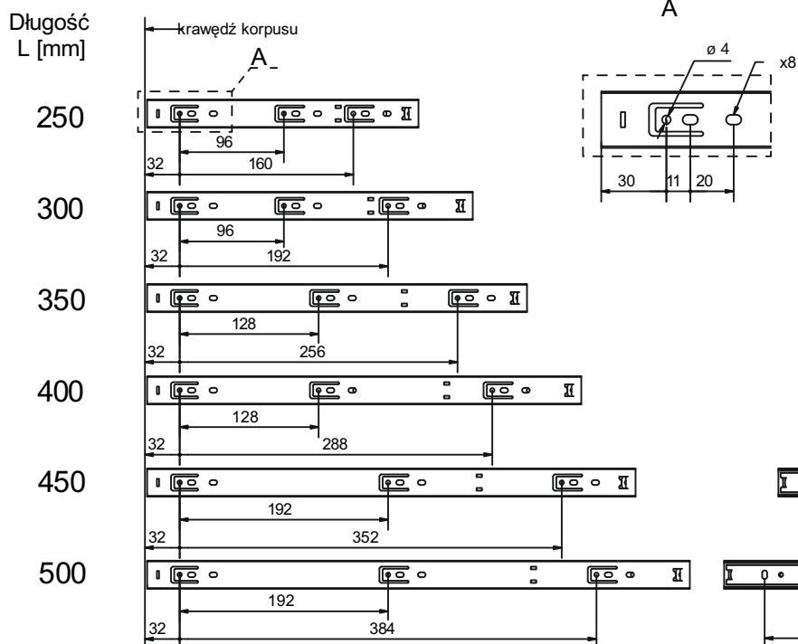
Widok na boku korpusu
