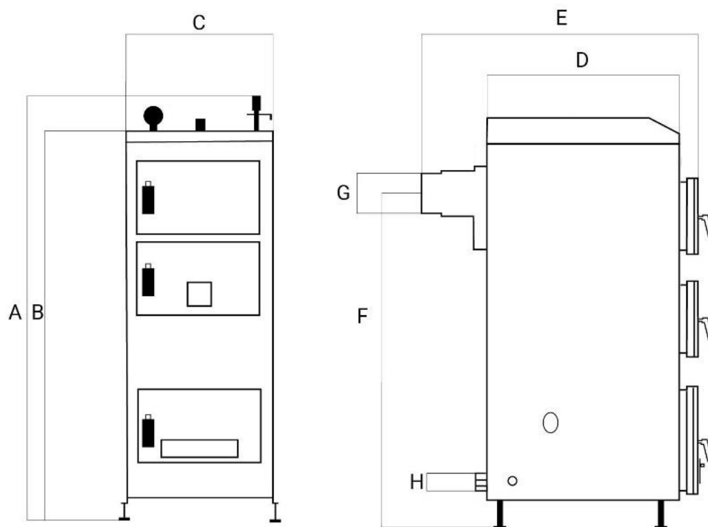
Rysunek 2. Wymiary kotła EKO UKS (w cm).
