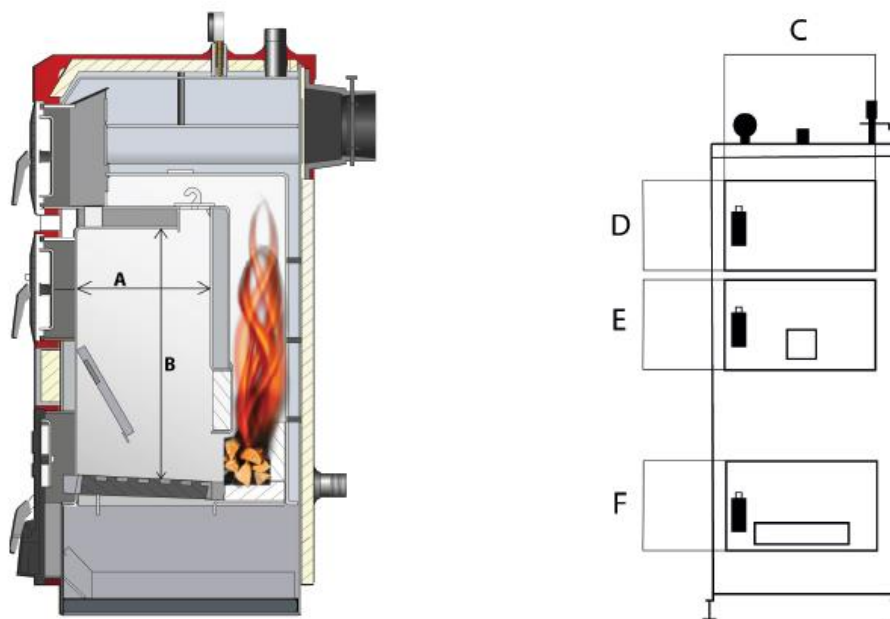
Rysunek 3. Wymiary paleniska i drzwi kotła EKO UKS (w cm).
