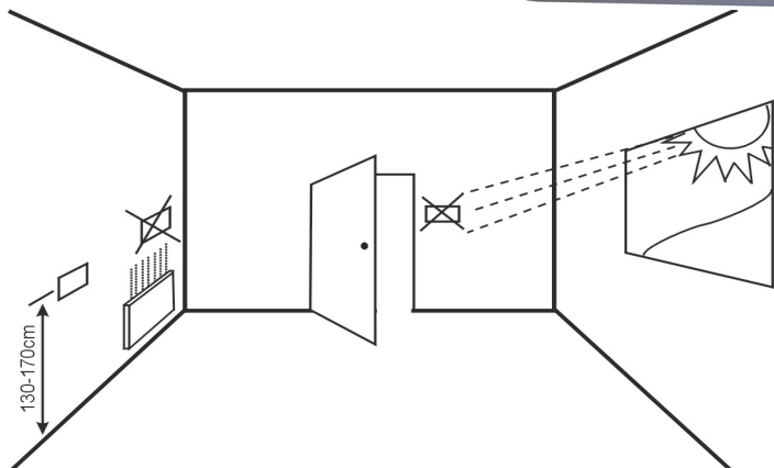
Rys. Prawidłowe umiejscowienie regulatora w pomieszczeniu.
