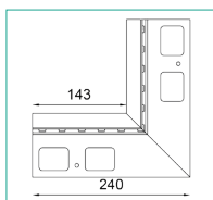
NAROŻNIK WEWNĘTRZNY K102 90
