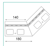
NAROŻNIK WEWNĘTRZNY K102 135
