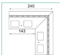
NAROŻNIK ZEWNĘTRZNY K102 90
