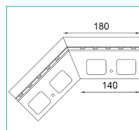
NAROŻNIK ZEWNĘTRZNY K102 135
