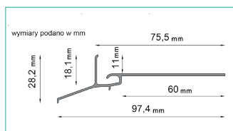
PROFIL OKAPOWY K102
