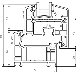
Przekrój poprzeczny Okno MDK De Luxe 70 o głębokości zabudowy 70 mm
