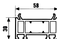
Poszerzenie ramy 3 cm
