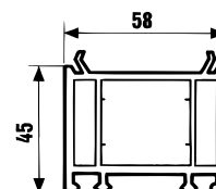
Poszerzenie ramy 4,5 cm
