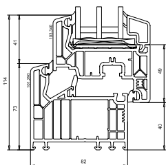
Przekrój poprzeczny Okno MDK De Luxe 82 o głębokości zabudowy 82 mm
