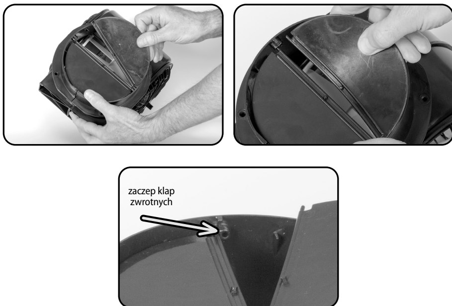
Ryc. 4. Montaż klap zwrotnych na wylocie turbiny
