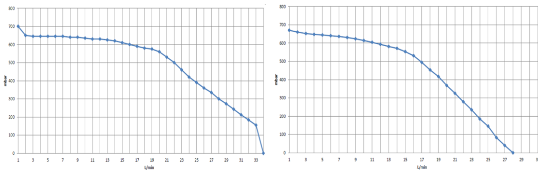
Rysunek 10: Wykresy natężenia przepływu przez obieg pierwotny (z lewej) i obieg grzewczy (z prawej) zestawu separacyjnego AHB 642 z zaworem termostatycznym ATV 213 i zaworem przełączającym AZV 643
