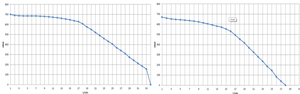
Rysunek 9: Wykresy natężenia przepływu przez obieg pierwotny (z lewej) i obieg grzewczy (z prawej) zestawu separacyjnego AHB 622 z zaworem termostatycznym ATV 213
