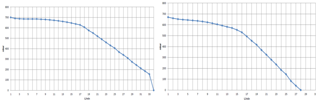
Rysunek 8: Wykresy natężenia przepływu przez obieg pierwotny (z lewej) i obieg grzewczy (z prawej) zestawu separacyjnego AHB 620
