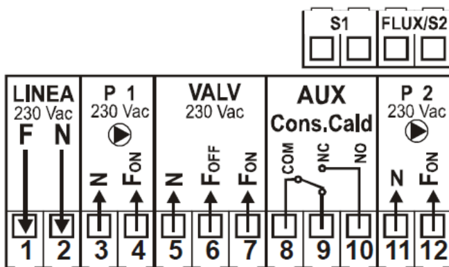
Rysunek 14: Przyłącza elektryczne zestawów separacyjnych AHB gdzie podłączane są:
