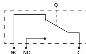
NVS 5 - Styk przełączny
