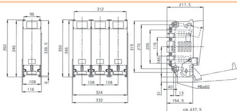
Rysunek wymiarowy rozłączników LTL4...
