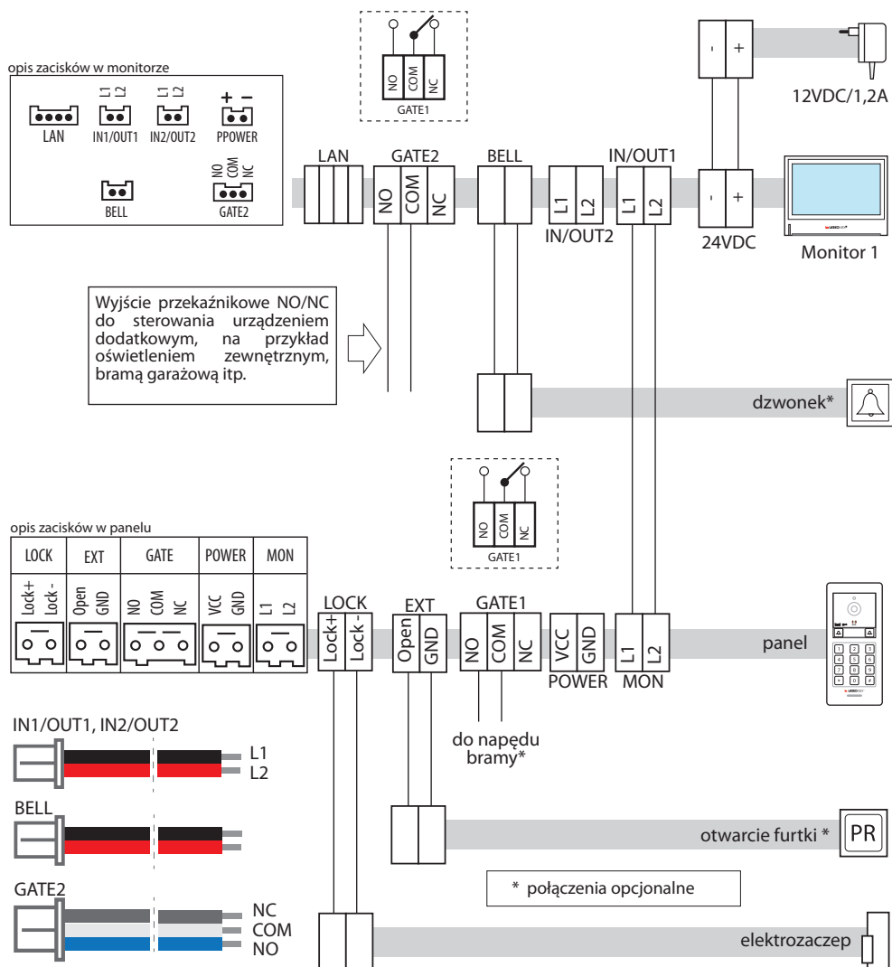
Rys. 9.1. Schemat połączeń - system podstawowy.
