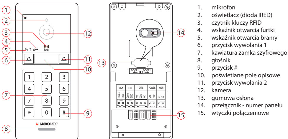
Rys. 3.2 Panel zewnętrzny.
