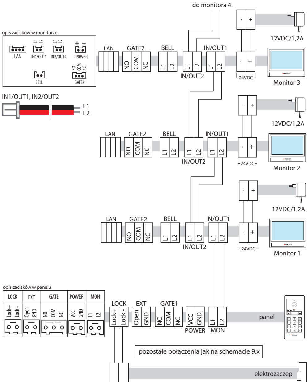
Rys. 9.5. Schemat połączeń- system z wieloma monitorami (max. 4).
