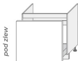
D1ZA 80 (800/820/500)
