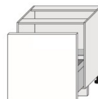
D1Z 80 + SEGREGO (800/820/500)
