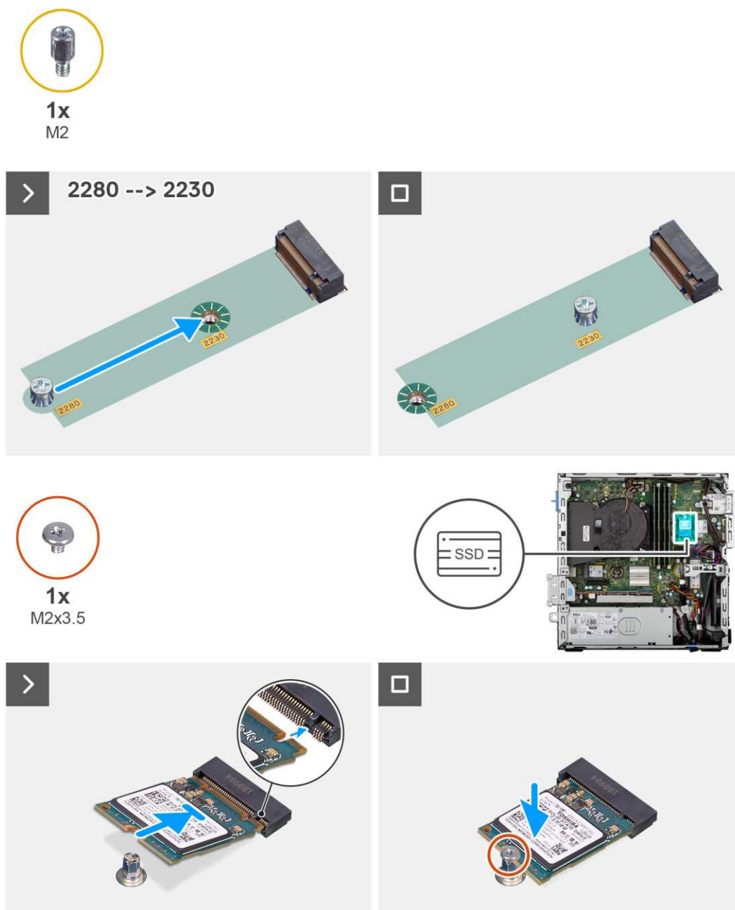
Rysunek 18. Instalowanie dysków SSD M.2 2230
