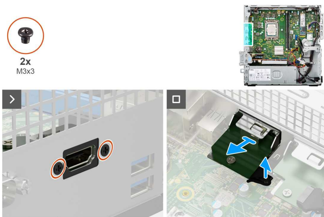
Rysunek 54. Wymontowywanie modułu złącza HDMI
