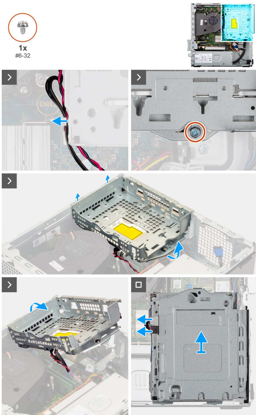
Rysunek 11. Wymontowywanie obudowy napędów
