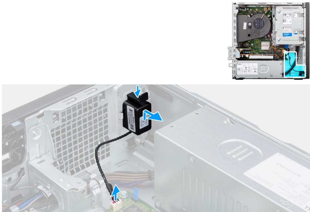
Rysunek 31. Wymontowywanie głośnika
