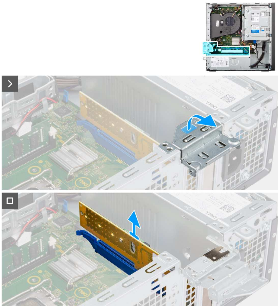
Rysunek 21. Wymontowywanie karty Dell Ultra Speed Drive trzeciej generacji
