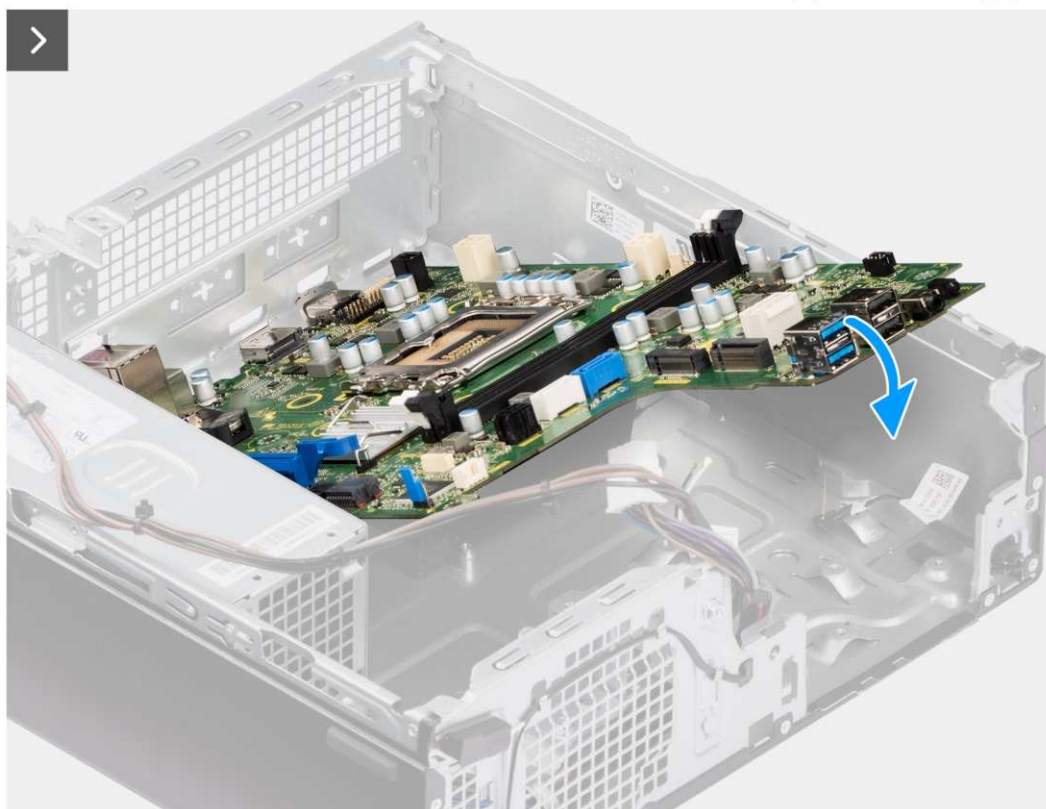
Rysunek 62. Instalowanie płyty głównej
