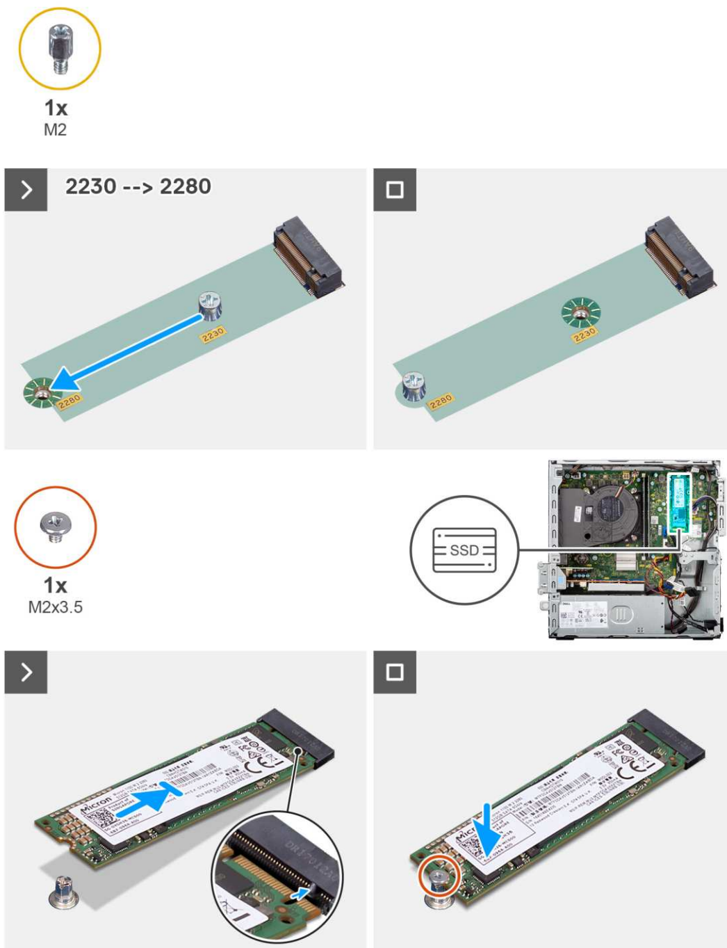
Rysunek 20. Instalowanie dysku SSD M.2 2280
