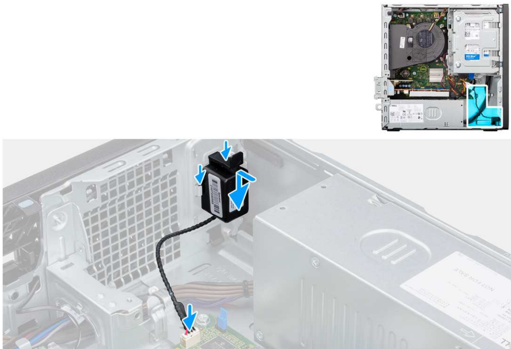
Rysunek 32. Instalowanie głośnika
