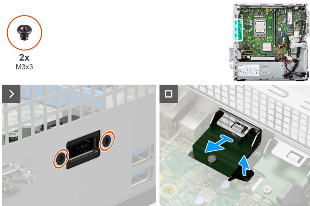
Rysunek 52. Wymontowywanie modułu DisplayPort
