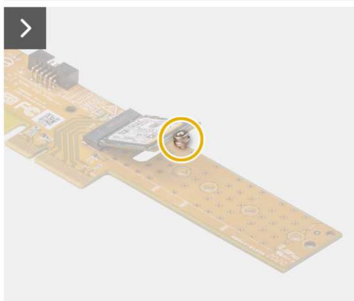
Rysunek 22. Wymontowywanie dysku SSD M.2 2230 z karty Dell Ultra Speed Drive trzeciej generacji
