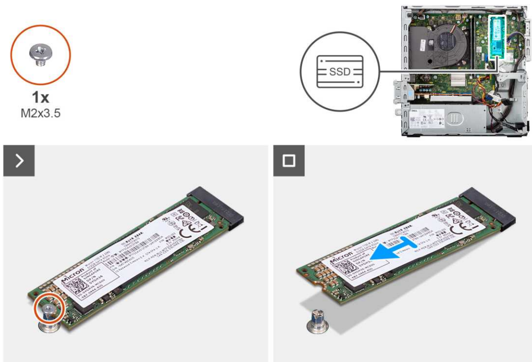
Rysunek 19. Wymontowywanie dysku SSD M.2 2280
