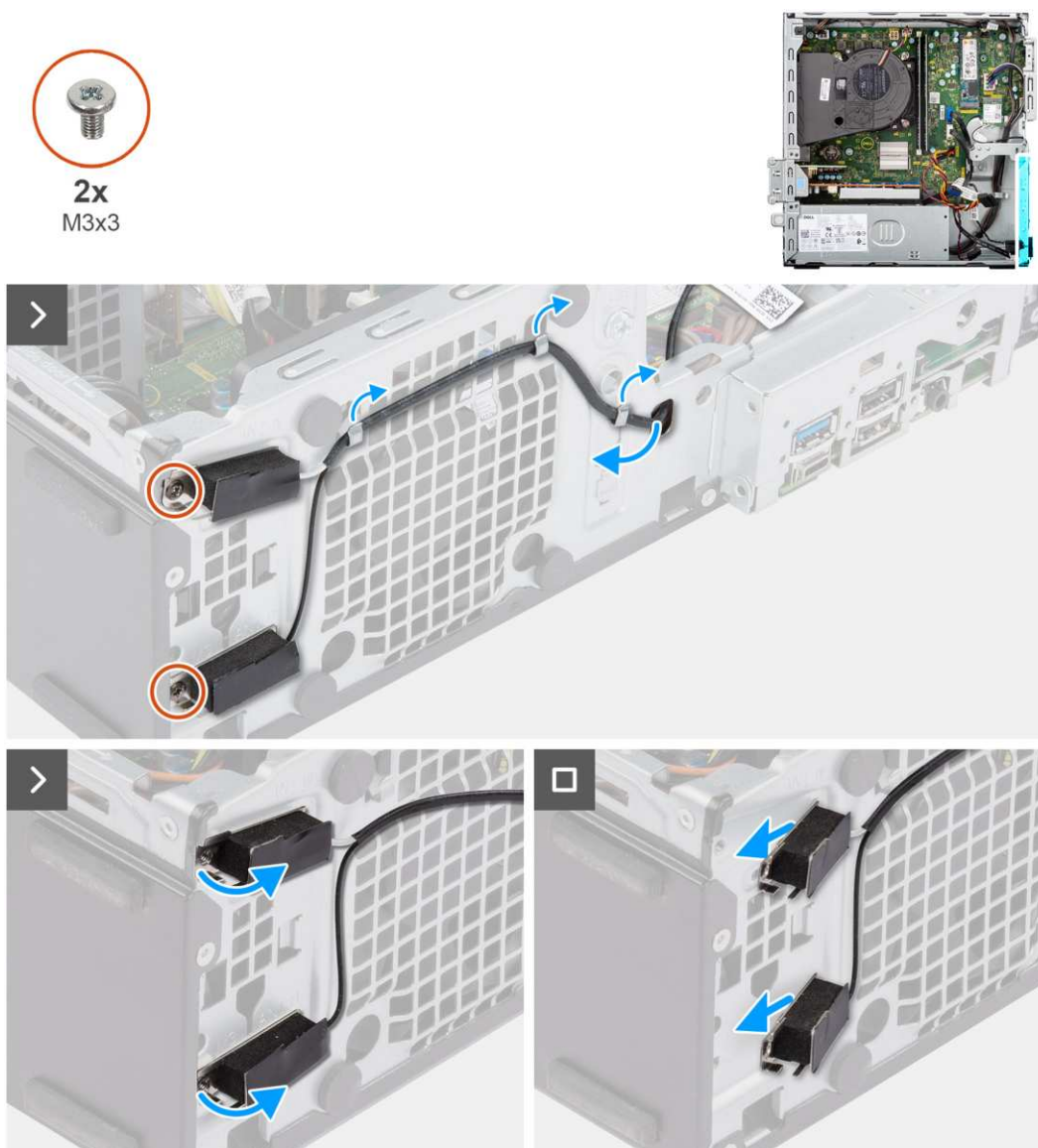
Rysunek 37. Wymontowywanie modułu anteny wewnętrznej
