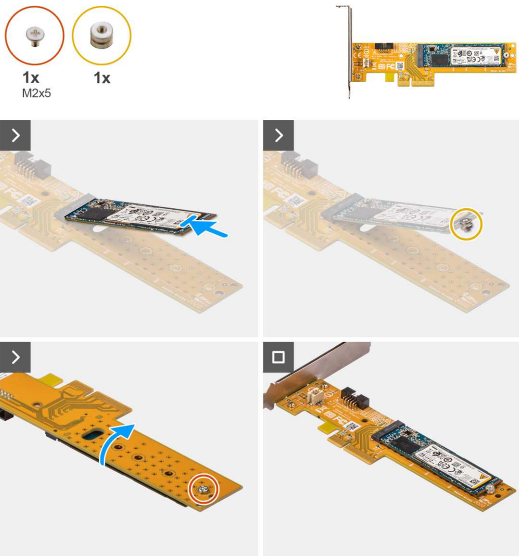
Rysunek 25. Instalowanie dysku SSD M.2 2280 na karcie Dell Ultra Speed Drive trzeciej generacji
