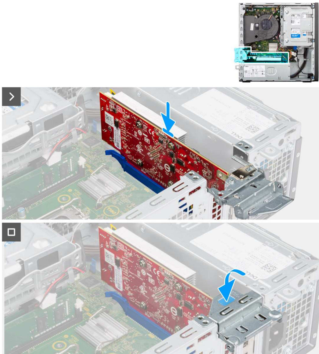
Rysunek 30. Instalowanie karty graficznej
