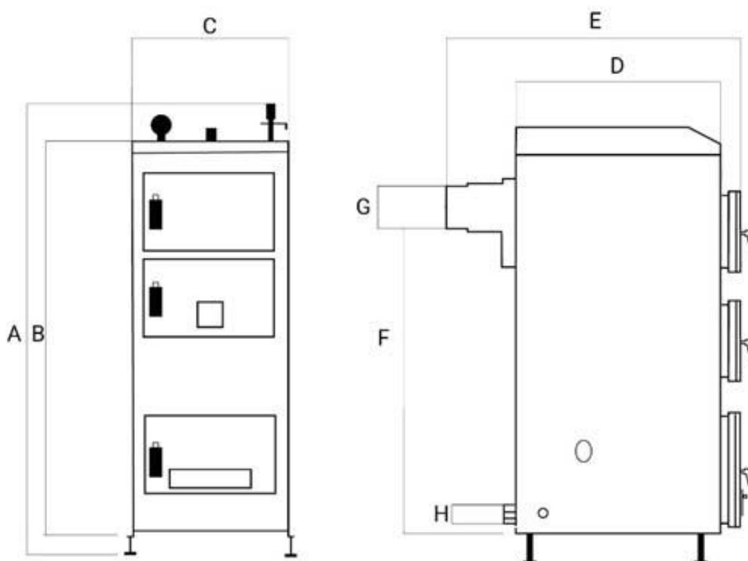
Rysunek 2. Wymiary kotła EKO UKS PLUS 2 (w cm).
