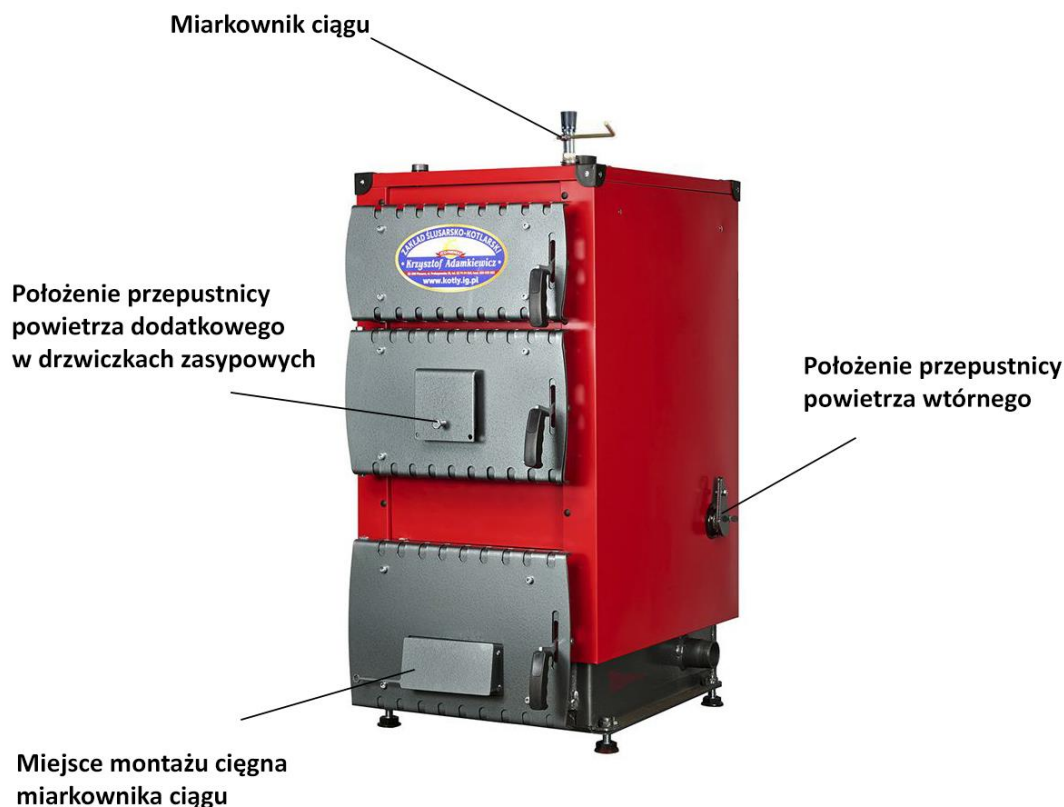
Rysunek 9. Metoda regulacji dysz powietrznych kotła.
