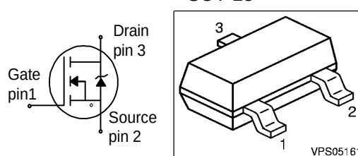
SOT-23
