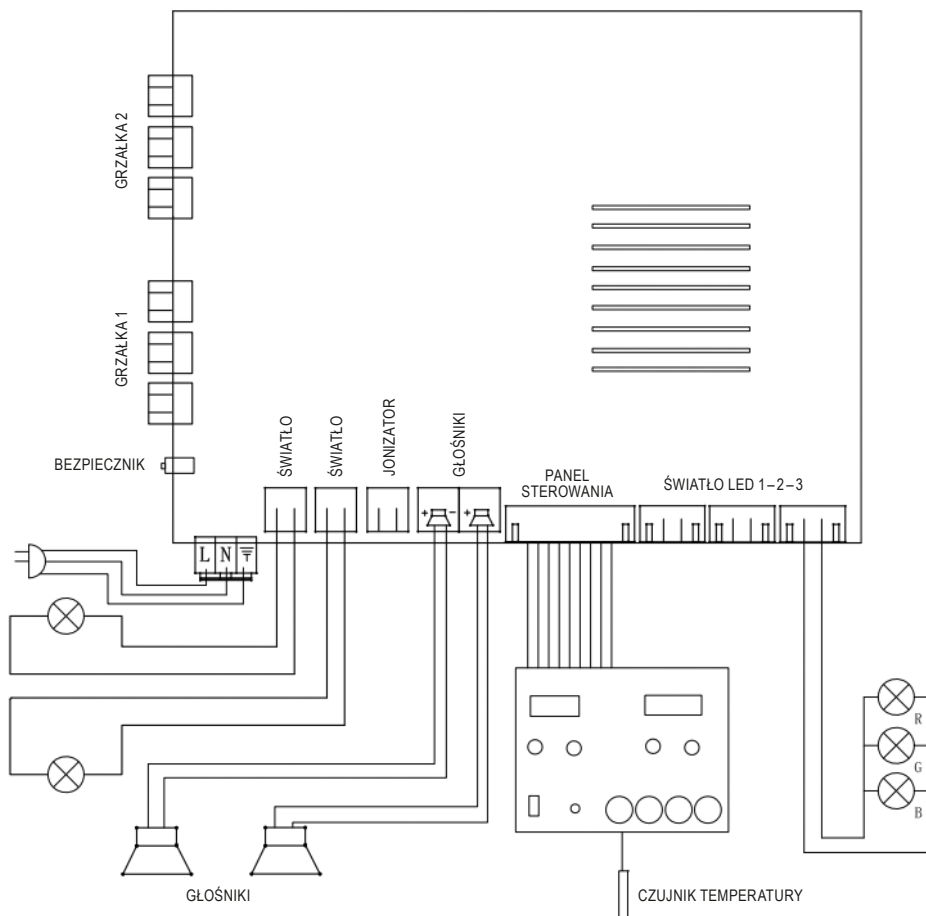
Rys. Schemat instalacji elektrycznej w saunie infrared.
