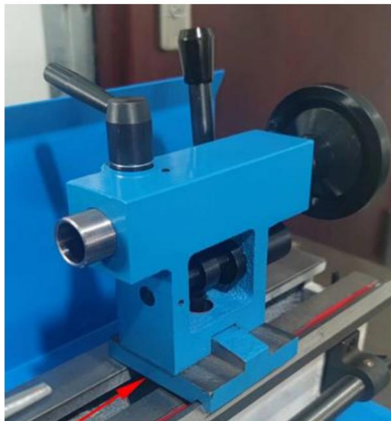
Rys. 3 Regulacja podpórki konika
