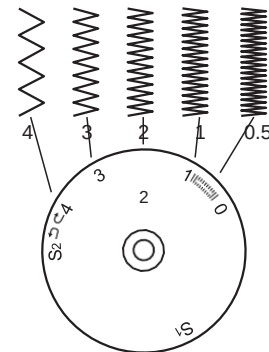
Pokrętło długości ściegu
