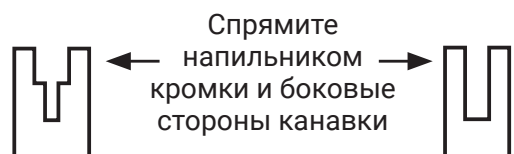
Изношенная канавка
