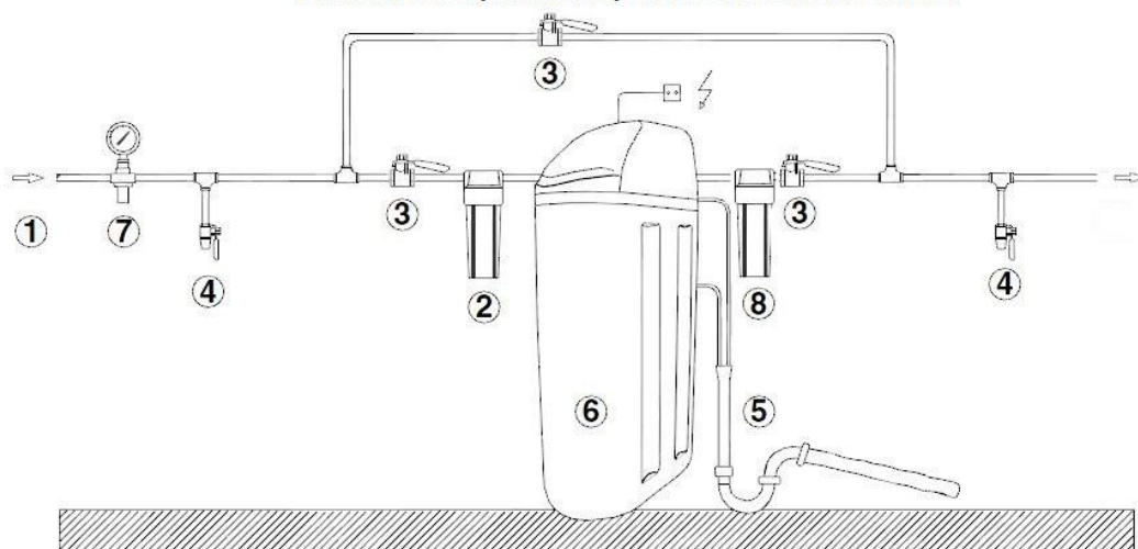
SCHEMAT PODŁĄCZENIA ZMIĘKZACZA / UZDATNIACZA WODY
