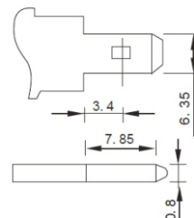
Złącze akumulatora
