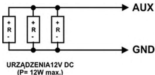
17 Sposób podłączenia dodatkowych urządzeń do wyjścia AUX.
