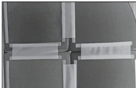
Sicherheitsorientiertes Klettverschluss-Design
