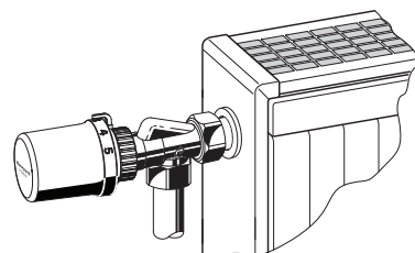
Rys. 3. Zawór osiowy
