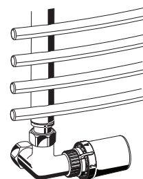
Rys. 6. Zawór narożny lewy zamontowany na grzejniku łazienkowym
