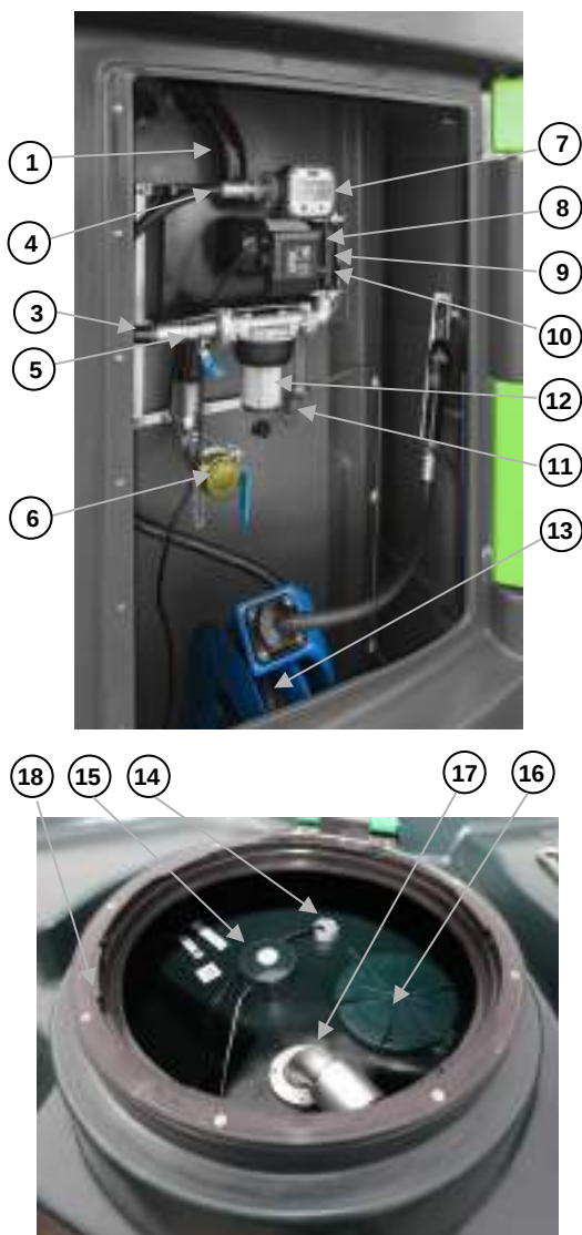
Widok po otwarciu pokrywy rewizyjnej urządzeń o pojemności 5000 l i powyżej.
