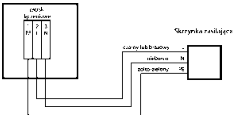
Schemat podłączenia elektrycznego urządzenia z rozdzielnią główną w układzie zasilania TN-S
