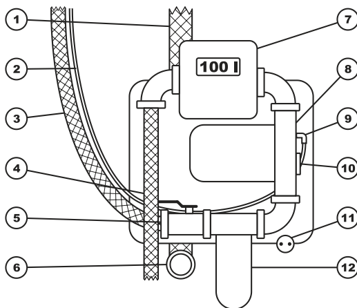
Schemat urz dzenia po otwarciu dystrybutora o pojemnoœci 3500 l i powyŹej.
