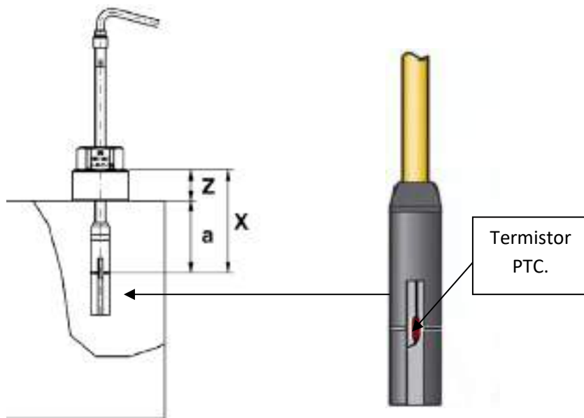
Sonda maksymalnego poziomu - elektroniczne zabezpieczenie.
