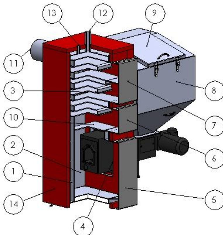
Rys.1. Kocioł "Technix (Dragon V Plus)"
