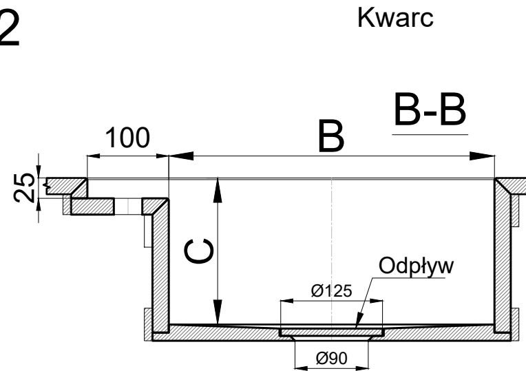
Zlewozmywak QSS02 (Zmienne wymiary w milimetrach)
