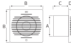
ÖLÇÜLER / DIMENSIONS
