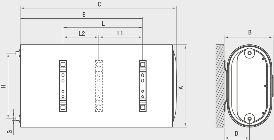
Montaż poziomy
