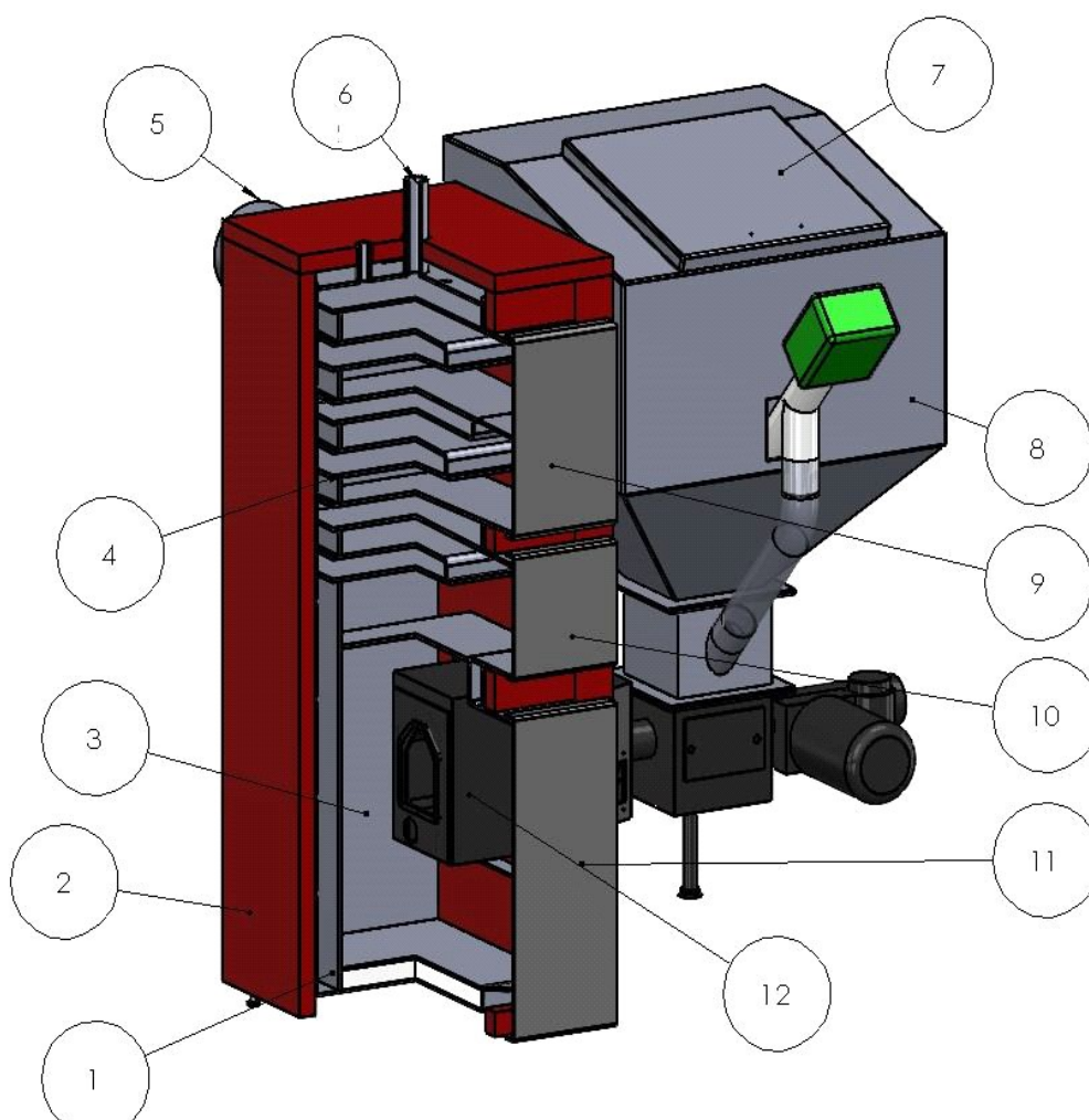
Rys.1. Kocioł "DRAGON V PLUS-PEL"
