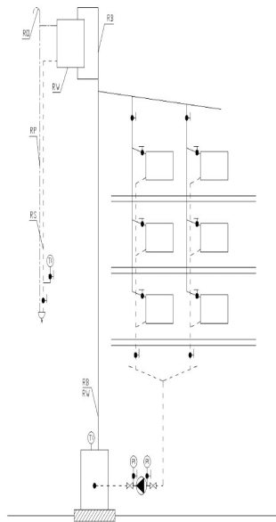
Rysunek 1b Schemat zabezpieczenia instalacji ogrzewania wodnego, wyposażonej w jeden kocioł lub wymiennik ciepła, rozdziel górny, pompa zamontowana na powrocie wg PN-91/B-02413
