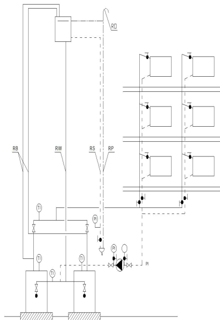
Rysunek 1c Schemat zabezpieczenia instalacji ogrzewania wodnego, wyposażonej w dwa lub więcej kotły lub wymienniki ciepła, rozdziel górny, pompa zamontowana na powrocie wg PN-91/B-02413
