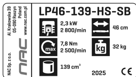
Tabliczka znamionowa
