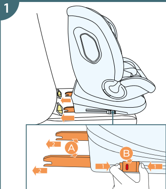
A: Ramiona ISOFIX B: Dźwignia zwalniająca ISOFIX
