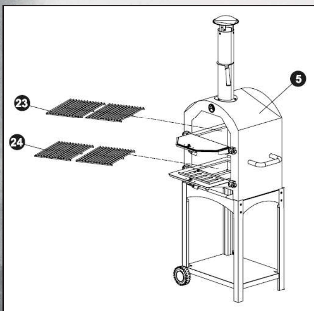
5. firebox 23. grill gratings 24. charcoal gratings 5. Popelník 23. Grilovací rošty 24. Rošty na dřevěné uhlí
