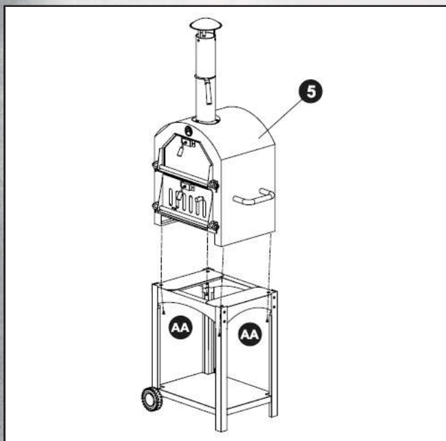
5. firebox 5. Ohniště
