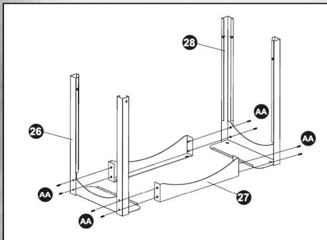
26. Podstavec s kolečky 27. Boční podpora 28. Část podstavce bez koleček 26. foot part with wheels 27. side support 28. foot part without wheels
