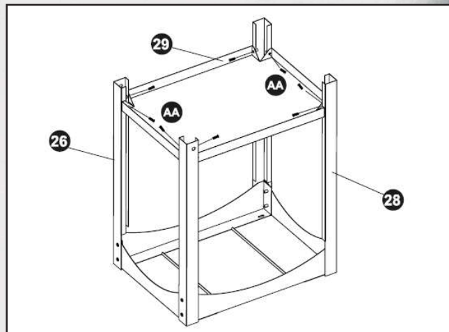
26. Podstavec s kolečky 28. Část podstavce bez koleček 26. foot part with wheels 28. foot part without wheels 29. Spodní deska
