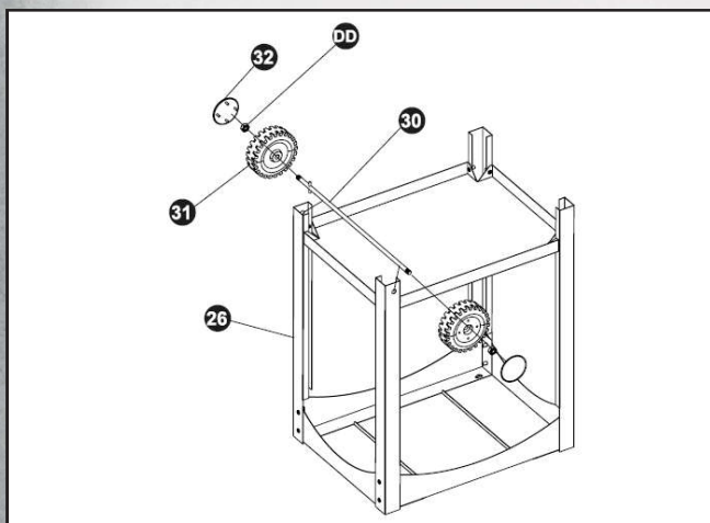
26. Podstavec s koly 30. Náprava 31. Kolo 32. Kryt kola 26. foot part with wheels 30. axle 31. wheel 32. wheel cap
