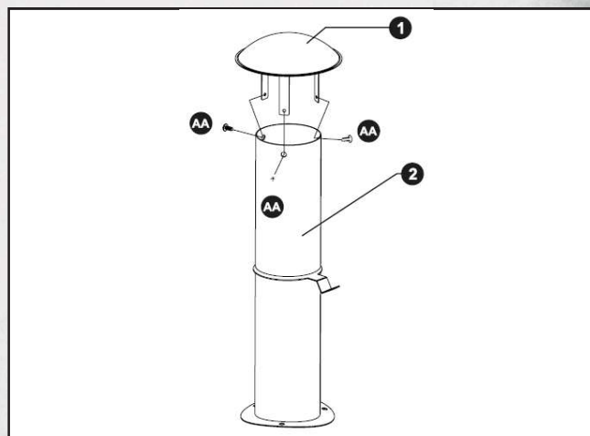
1. Ochrana proti dešti 2. Komin 1. rain cap 2. chimney
