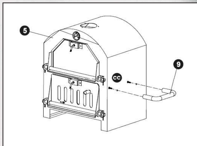
5. Ohniště 9. Držadlo 5. firebox 9. handle
