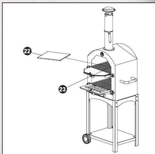
22. pizza stone 23. grill gratings 22. Pizza kámen 23. Grilovací rošty
