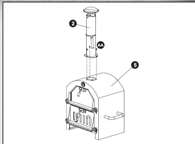
2. Komin 5. Ohniště 2. chimney 5. firebox
