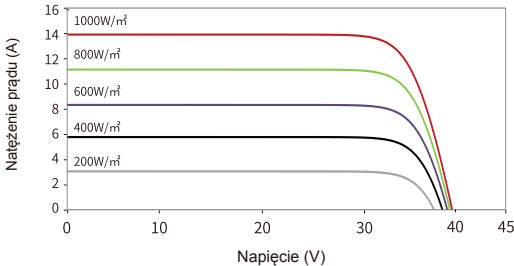
Wykres prądu w funkcji napięcia (54HL4R-(V) 450W)
