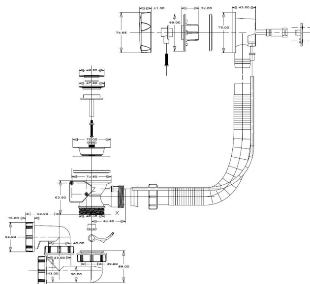
rysunek techniczny
