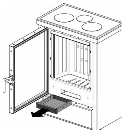
3. Następnie wyjąć szufladę na popiół
