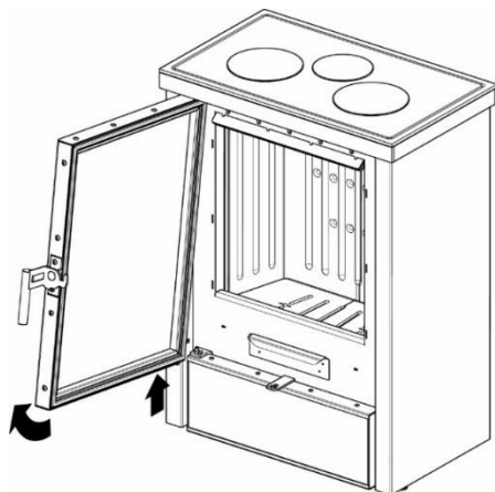
Rysunek 9. Demontaż drzwi ogrzewacza
