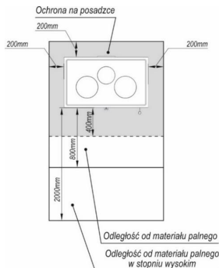
Rysunek 3. Minimalne bezpieczne odległości przy ustawianiu ogrzewacza.
