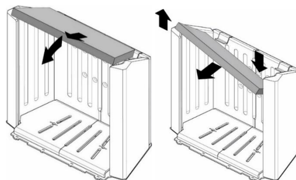
Rysunek 10. Demontaż deflektora
