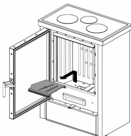
2. Wyjąć jedną część rusztu
