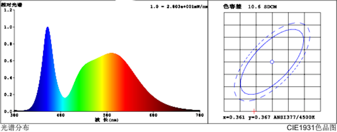
光谱分布
